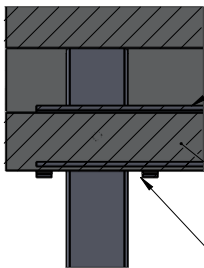
Single layer of FyreWrap®
